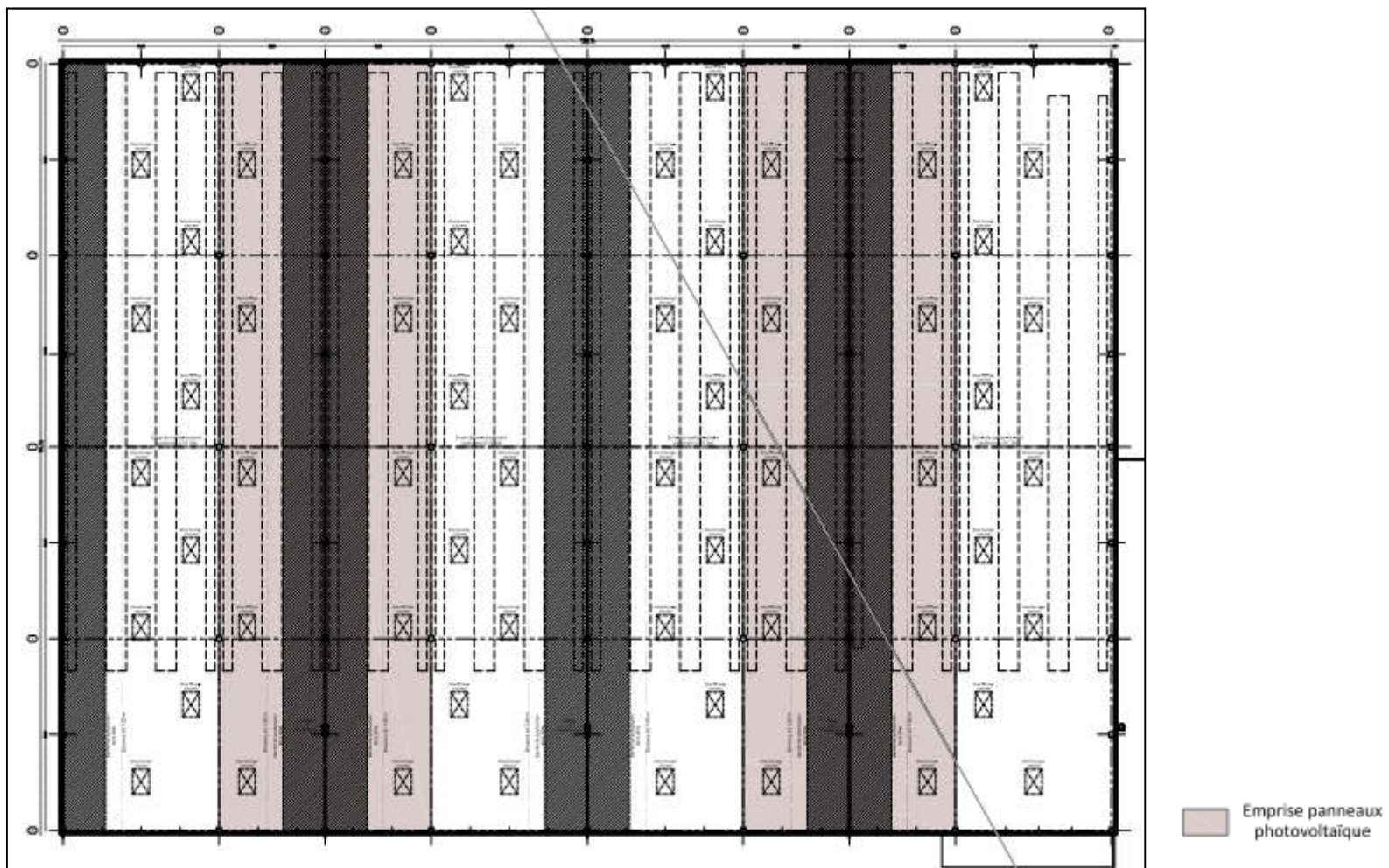
Plan d'implantation prévisionnel de l'emprise des panneaux photovoltaïques : ce plan de principe ne tiens pas compte des reculs avec les exutoires qui seront respectés sur le plan définitif : un plan sera transmis à l'inspection des installations classées.
